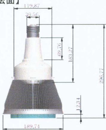
【寸法面】
